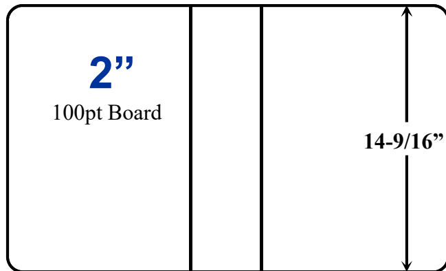
D-R SD Ring 11-1/4" 3-1/16" 11-1/4" Die # LB334
